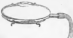
Fig. 93. — Appareil explorateur de la contraction des muscles thoraciques de l'oiseau. La face supérieure convexe est formée par la membrane de caoutchouc soulevée par le ressort-boudin; c'est elle qui s'applique sur les muscles. La face inférieure, en contact avec le corset, porte quatre petites griffes qui s'implantent dans l'étoffe et maintiennent l'appareil en place.
